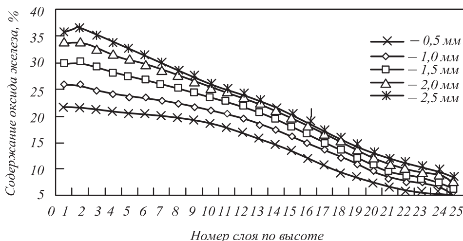
Рис. 6. Содержание оксида железа по высоте колонного реактора в зависимости от крупности частиц железной руды
