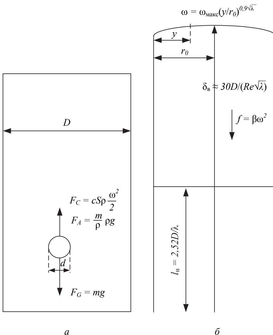
Рис. 3. Силы, действующие на частицу в гравитационном сепараторе (а); эпюра скоростей для турбулентного течения (б)
