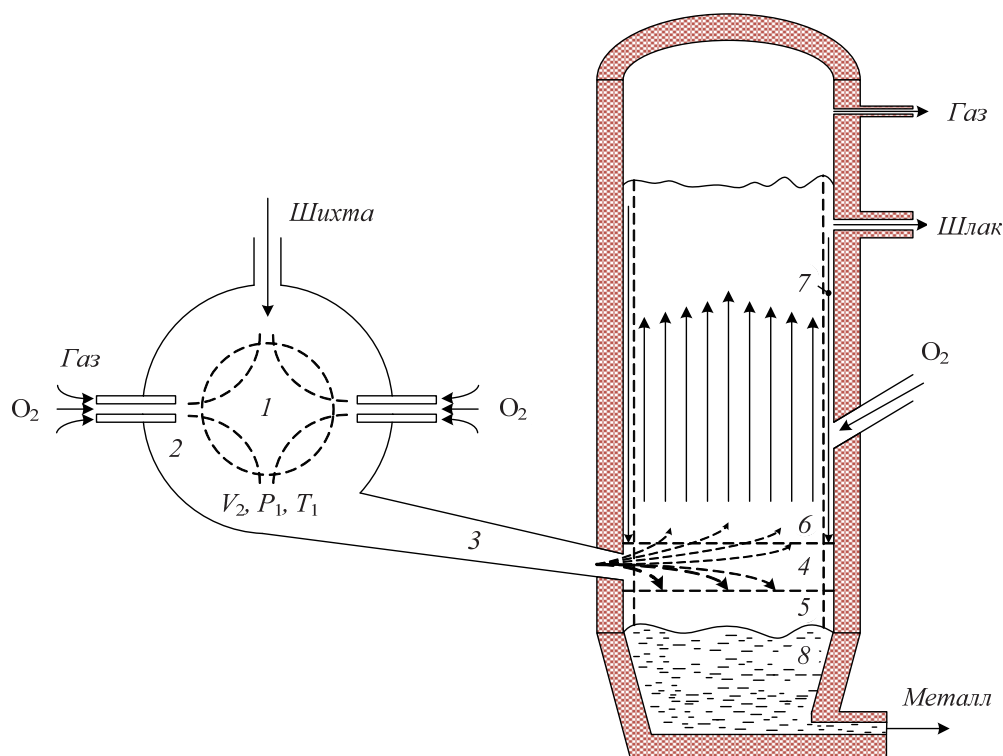
Рис. 2. Зонная модель процесса СЭР
