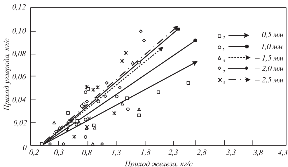
Рис. 7. Зависимость прихода углерода от прихода железа при различной крупности частиц железной руды
