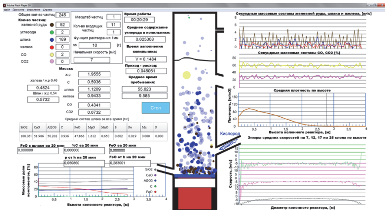
Рис. 4. Интерфейс программы имитационного моделирования
