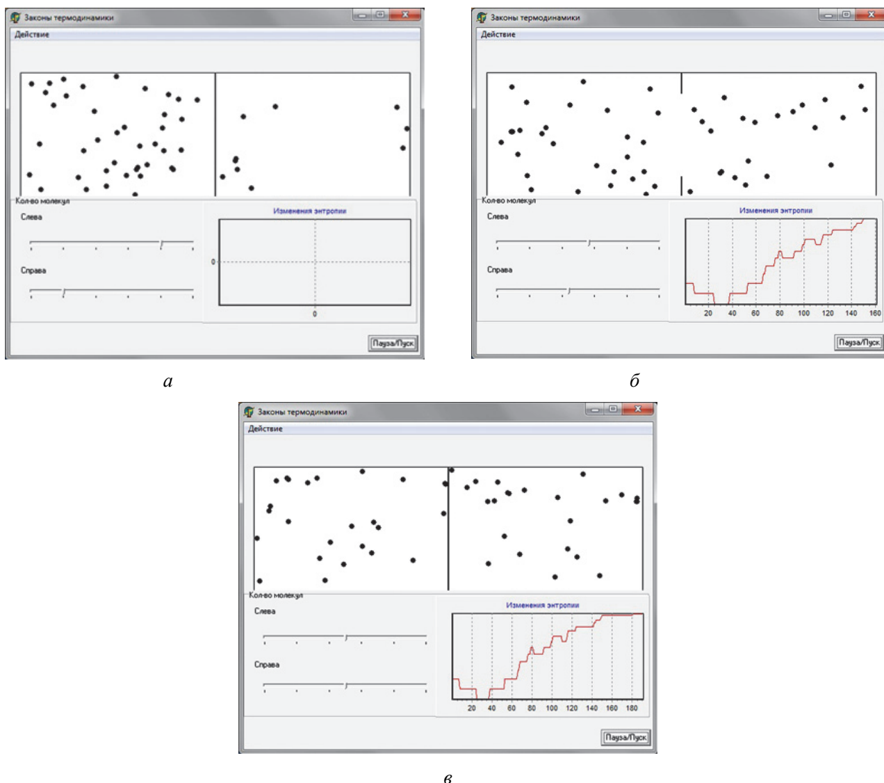
Рис. 1. Увеличение энтропии при смешении
