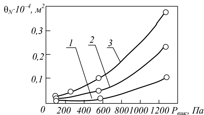
Рис. 4. Зависимость относительного количества структурных углублений напыленного слоя шихты от давления ВПС; уравнения регрессии для различной влажности шихты: 1 – W_{ш} = 5,5\% ( y = 0,0237e^{0,0023x} , R^2 = 0,9921 , y = \theta_N \cdot 10^{-4} , x = P_{впс} ); 2 – W_{ш} = 7,5\% ( y = 0,0163e^{0,0022x} , R^2 = 0,9996 ); 3 – W_{ш} = 9,5\% ( y = 0,0079e^{0,002x} , R^2 = 0,9801 )
