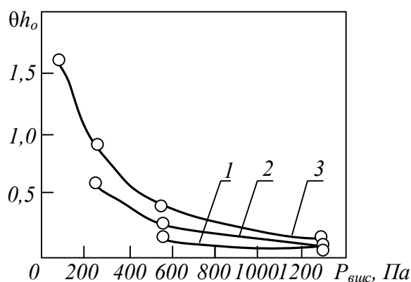
Рис. 3. Зависимость относительной величины структурных углублений от давления ВПС; уравнения регрессии для различной влажности шихты: 1 – W_{ш} = 5,5\% ( y = 1,878e^{-0,0024x} , R^2 = 0,9884 ; y = \theta_{ho} , x = P_{впс} ); 2 – W_{ш} = 7,5\% ( y = 0,9376e^{-0,0018x} , R^2 = 0,9925 ); 3 – W_{ш} = 9,5\% ( y = 0,3644e^{-0,001x} , R^2 = 1 )
