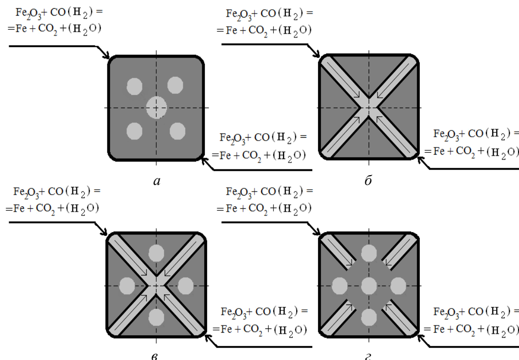
Рис. 1. Схемы различных вариантов реакционной способности брикетов в зависимости от вида пористости: а – закрытая труднопроницаемая для газов; б – открытая легкопроницаемая для газов; в, г – комбинированные варианты
