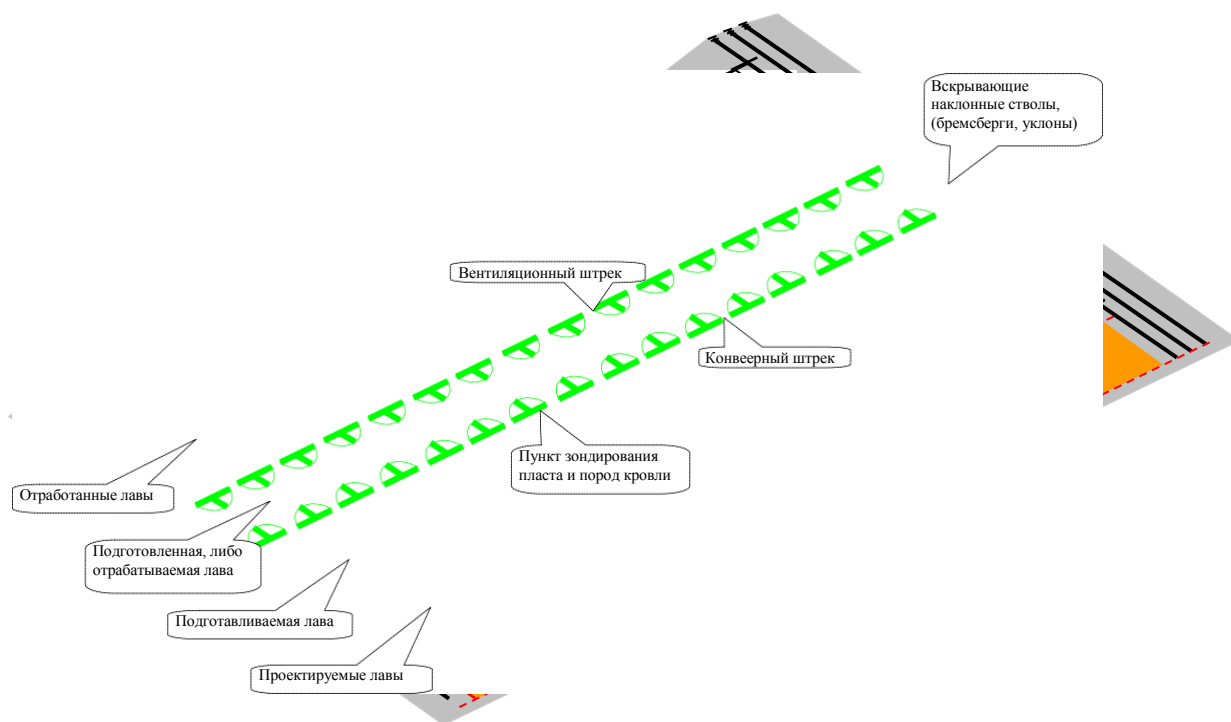
Типовая схема размещения пунктов геофизического мониторинга при оценке геомеханического состояния подготовленного или отрабатываемого выемочного участка с использованием аппаратуры бесконтактного зондирования типа АЭШ-1 [2]
