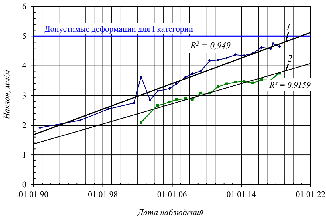
Рис. 6. Максимальные наклоны стволов "Северный" (1) и "Ново-Капитальный" (2) в этаже +390 ÷ +450 м
