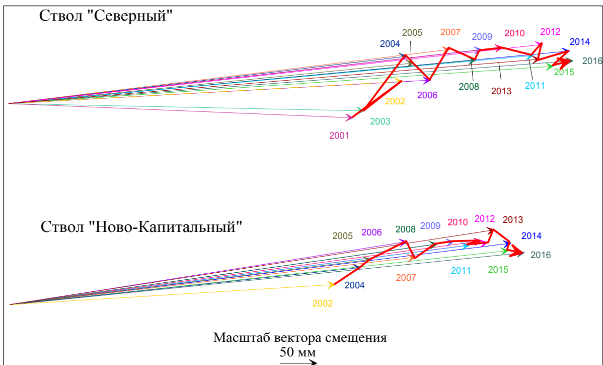
Рис. 4. Векторы максимальных смещений стволов на гор. +450 м
