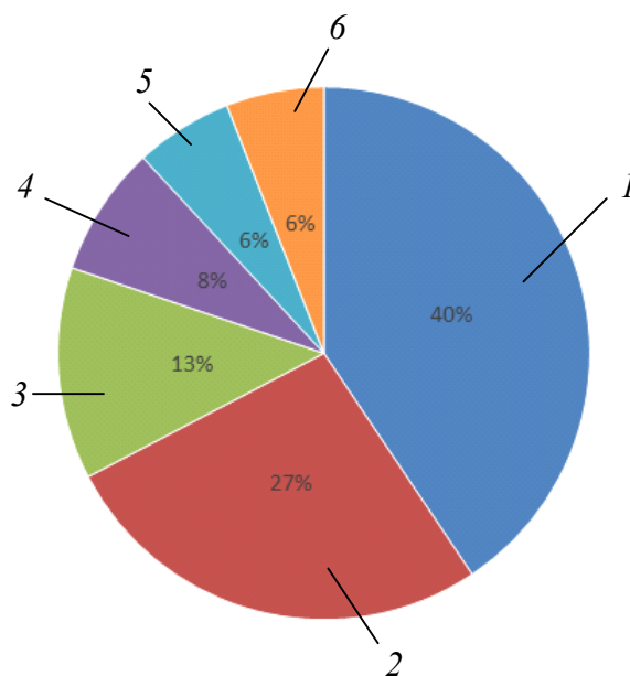
Рис. 2. Распределение простоев в проходческих забоях шахты «Распадская-Коксовая», октябрь 2016 г.: 1 – бурение профилактических скважин; 2 – превышение уровня CH 4 ; 3 – прочие организационные простои; 4 – ремонты оборудования; 5 – отсутствие электроэнергии; 6 – поломка ленточного конвейера
