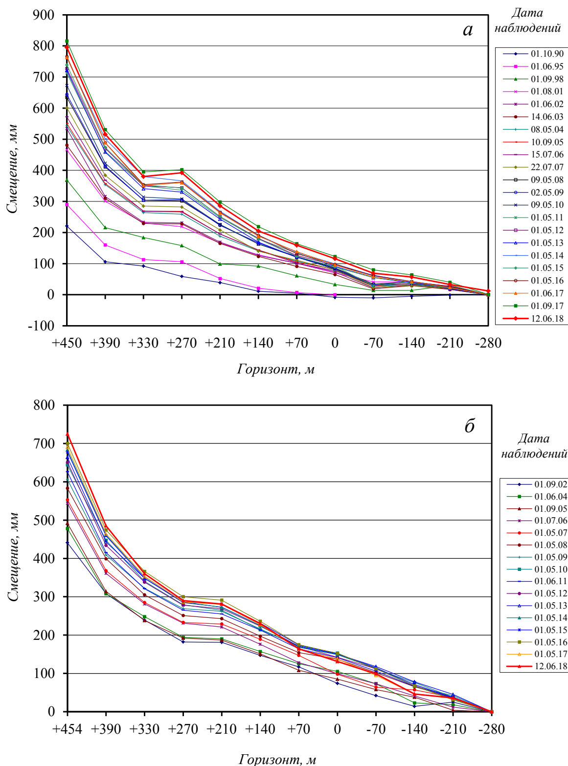
Рис. 2. Смещения стволов по горизонтам шахты в различные дни наблюдений: а – ствол «Северный»; б – ствол «Ново-Капитальный»
