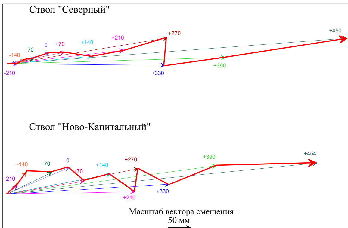
Рис. 5. Векторы смещения стволов по горизонтам шахты -210 \div +454 м
