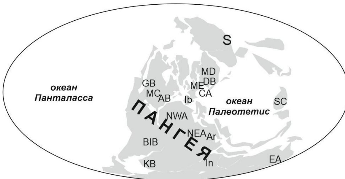
Рис. 2. Расположение изученных территорий в позднем палеозое. Глобальная реконструкция по К. Скотезе (Scotese, 2004)
