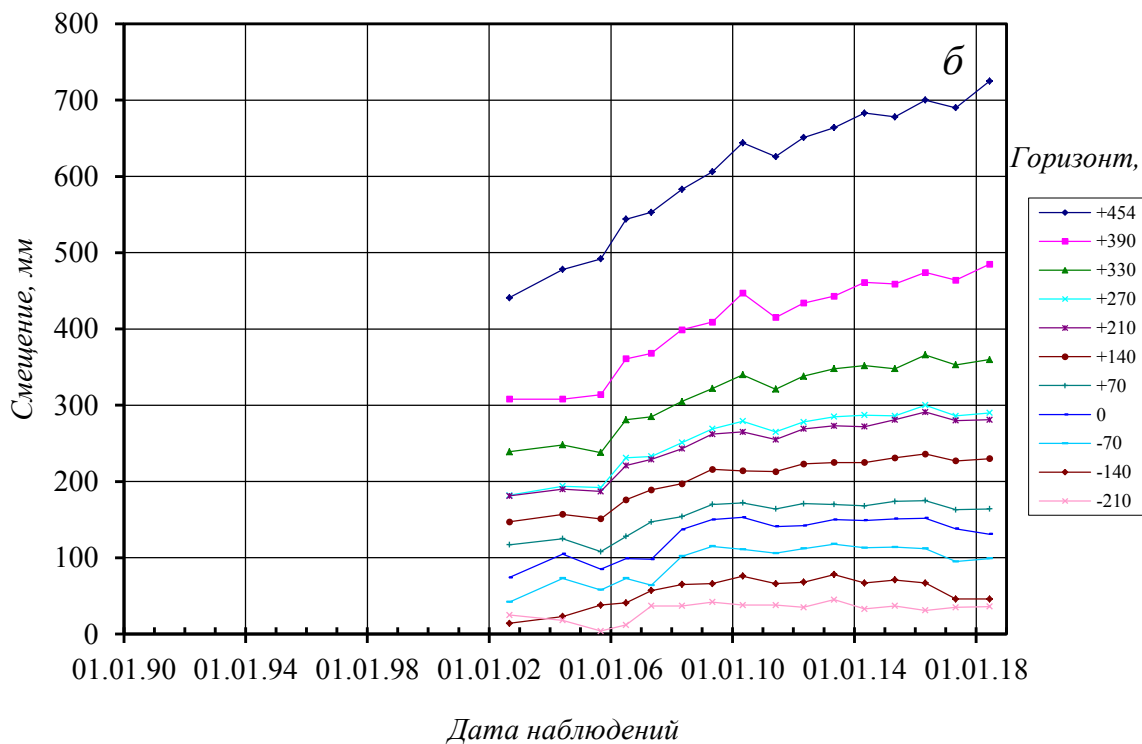
Рис. 3. Развитие во времени смещений стволов на горизонтах шахты а – ствол «Северный»; б – ствол «Ново-Капитальный»
