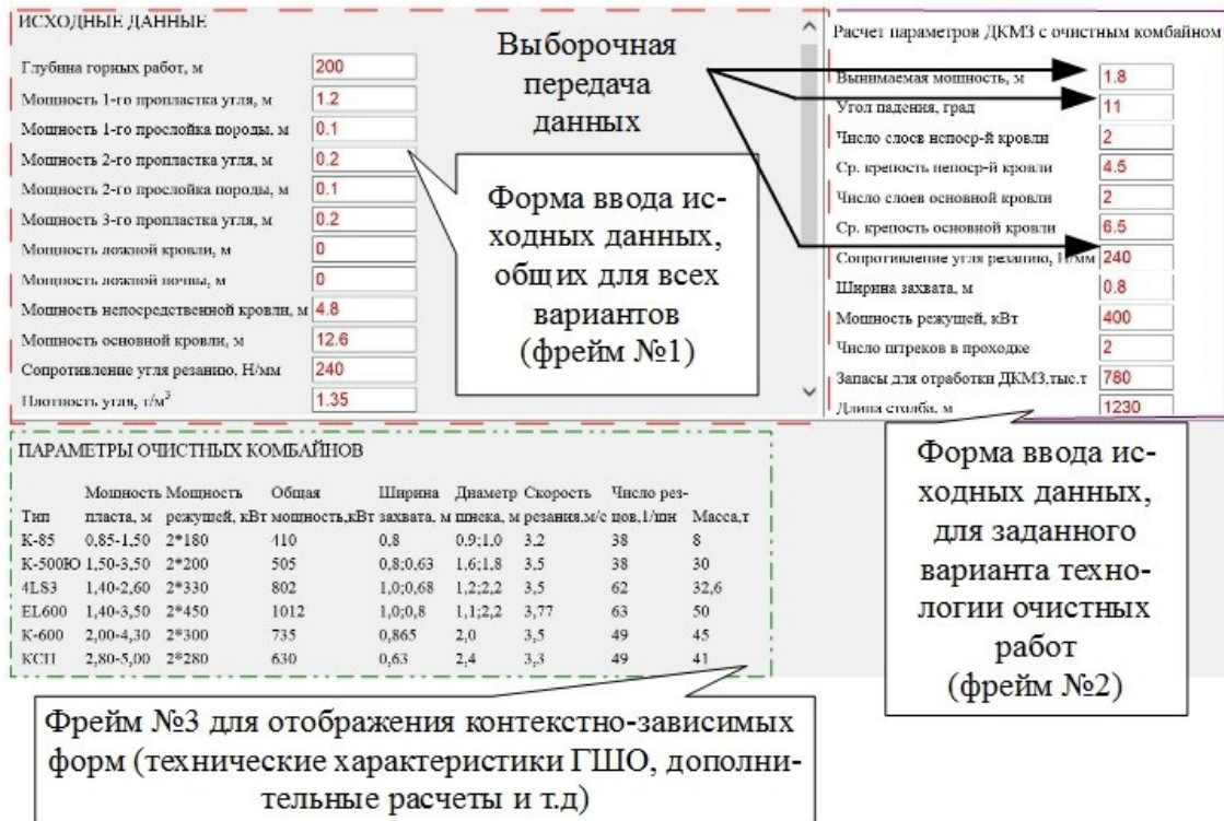
Рис. 1. Реализация интерфейса компьютерной лабораторной работы с использованием фреймов
