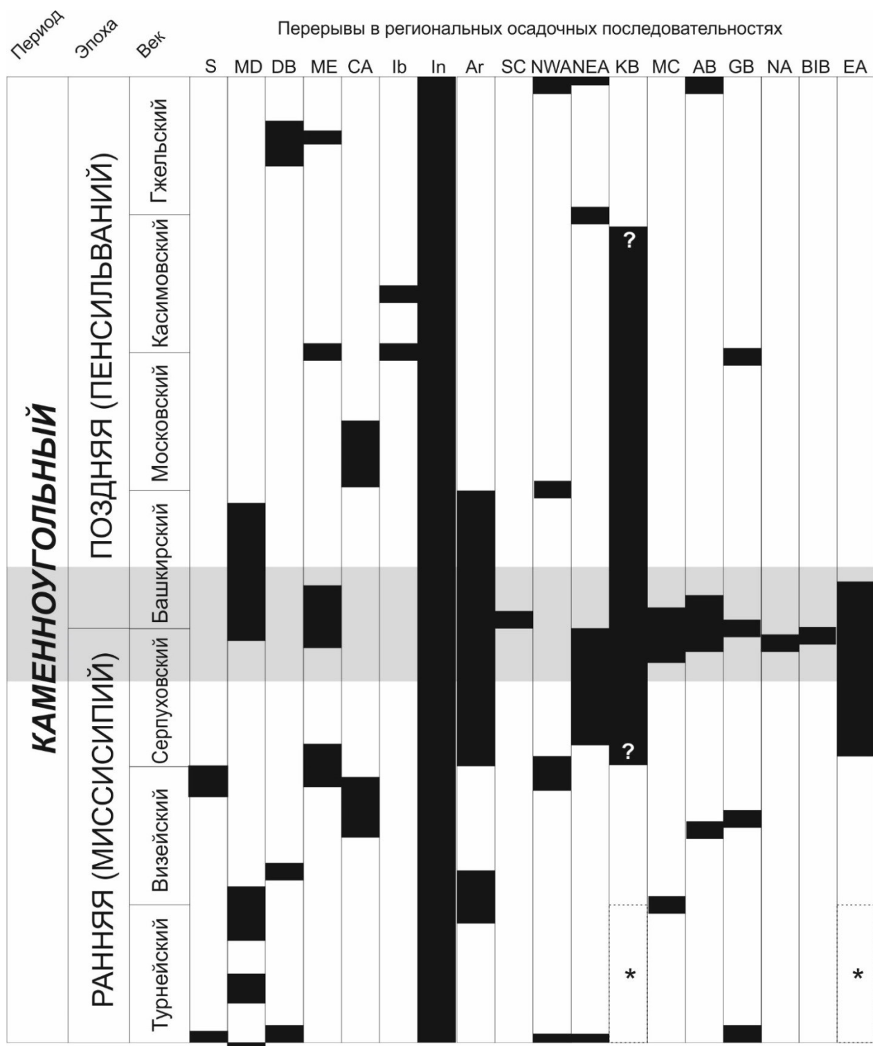
Рис. 1. Региональные перерывы каменноугольного периода. Серым показан квазиглобальный перерыв. Обозначения: АВ – Аппалачский бассейн, Аг – Аравийский полуостров, ВВВ – бразильские внутриконтинентальные бассейны, СА – Карнийские Альпы, DB – Донбасс, EA – Восточная Австралия, GB – Великий бассейн, In – Индия, KB – бассейн Кару, MC – Мидконтинент, MD – Московская синеклиза, ME – Средняя Европа, NEA – Северо-Восточная Африка, NWA – Северо-Западная Африка, S – Южная Сибирь, SC – Южный Китай, (NA – Северная Америка в целом), * – отсутствие данных о турнейских отложениях, ? – предположительная длительность перерыва
