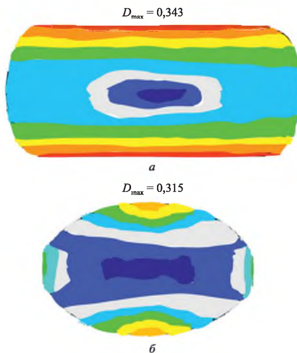
Рис. 2. Распределение критерия Кокрофта-Лэтэма по сечению раската при производстве сортовых заготовок диаметром 60 мм из отбраковки рельсовой стали марки К76Ф (табл. 1):
